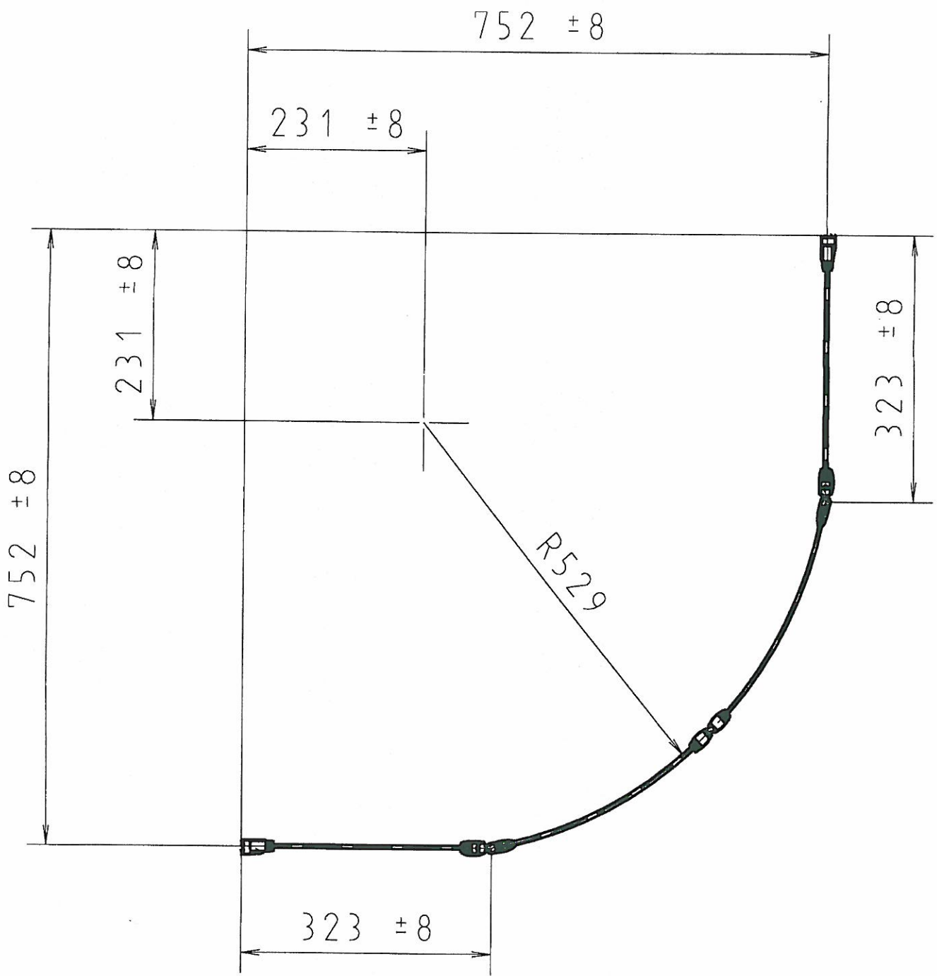
Runddusche D235004 Montage auf Fliesenfuge
